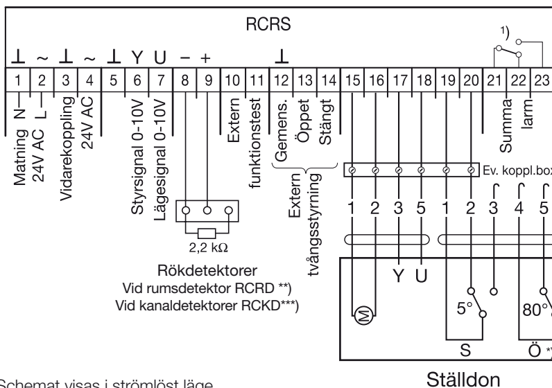
Schemat visas i strömlöst läge.
